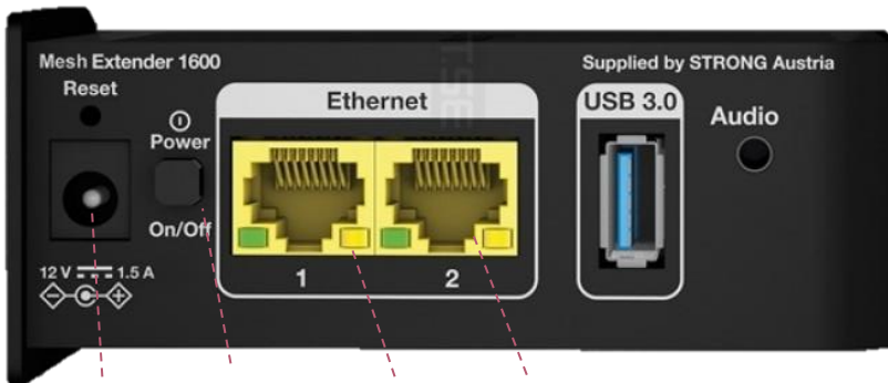
Strøm Tænd/Sluk LAN 1 LAN 2
